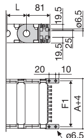
Fig. A Fissaggio della catena sull'esterno raggio. (Fig. A)
