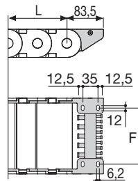
Fig. B Fissaggio della catena sull'esterno raggio. (Fig B)
