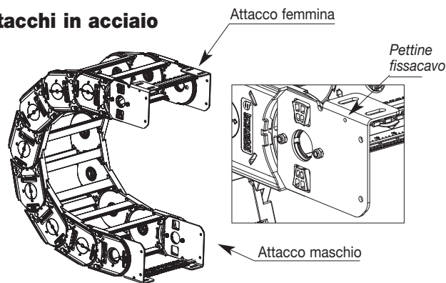
Fig. A Catena fissata sull'esterno raggio. (Fig A) Vedi varianti di montaggio a pag. 31.
