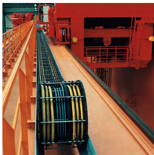
Catena tipo 318 per corse lunghe installata su carroponete.
