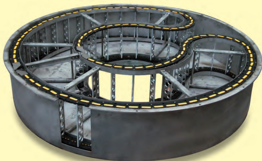
Rotazione in piano con due catene. Rotazione 370°.
