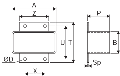
前端法兰型号 F1
